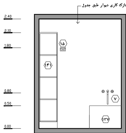
نقشه ۲-۲۴- نمای ۳- مقیاس ۱:۵۰
