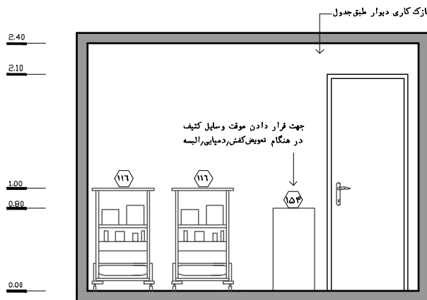
نقشه ۲-۳۷- نمای ۳- مقیاس ۱:۵۰
