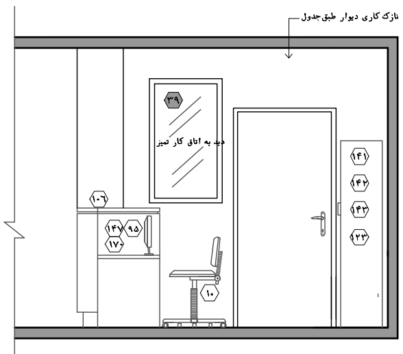
نقشه ۴-۵۵-۱- نمای ۴- مقیاس ۱:۵۰
