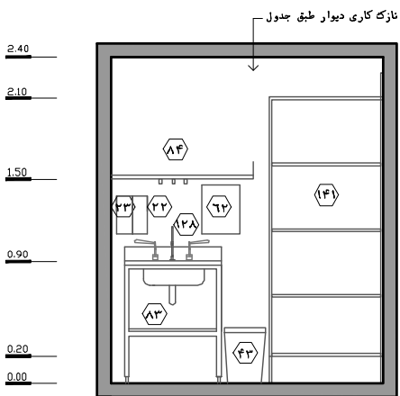
نقشه ۲-۲۳- نمای ۲- مقیاس ۱:۵۰
