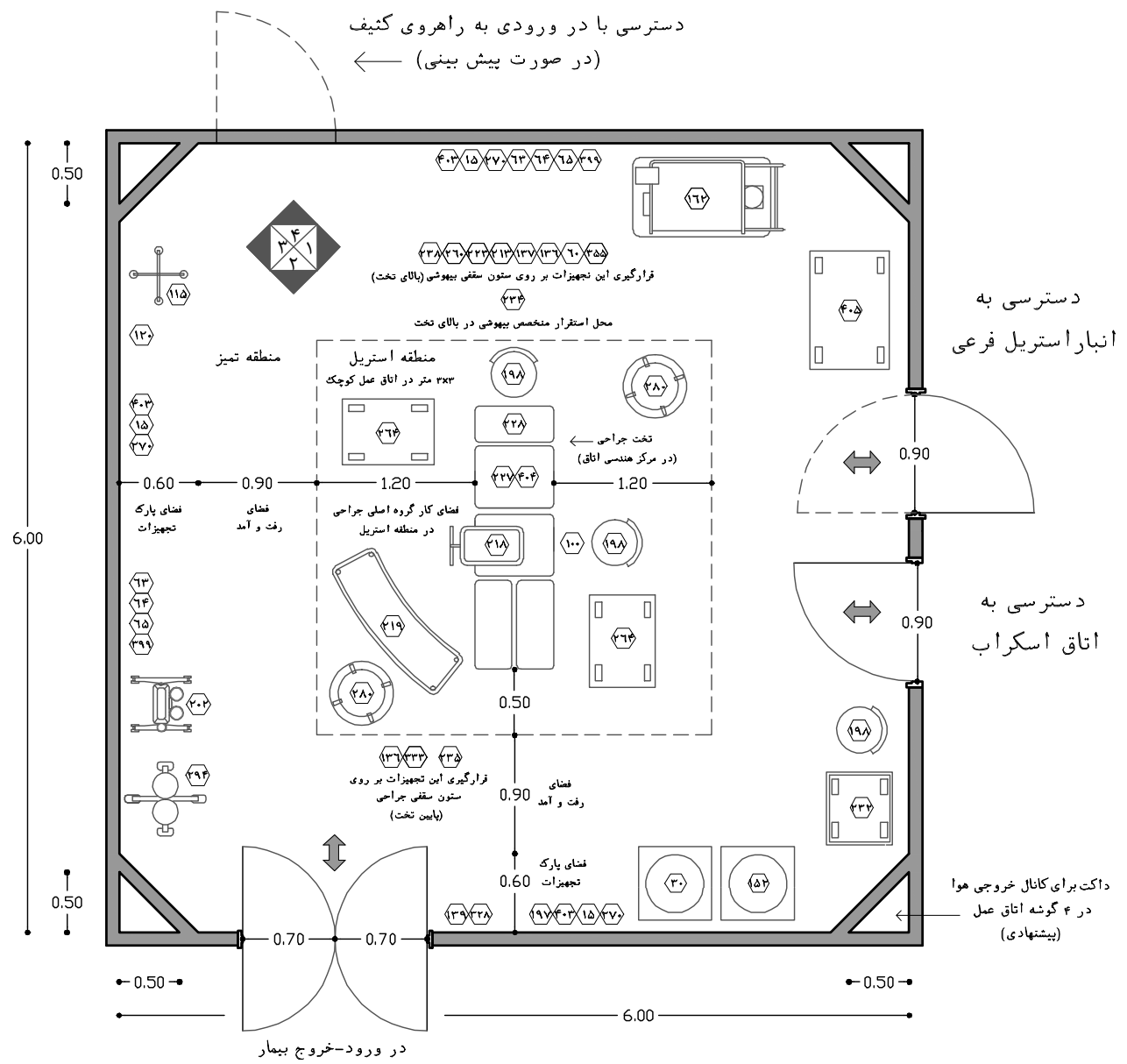
نقشه ۲-۱۴۵- پلان نمونه ای اتاق عمل جراحی کوچک - مقیاس ۱:۵۰
