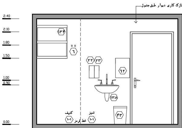
نقشه ۲-۳۵- نمای ۱- مقیاس ۱:۵۰
