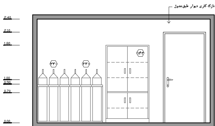
نقشه ۱۰۳-۲- نمای ۳- مقیاس ۱:۵۰
