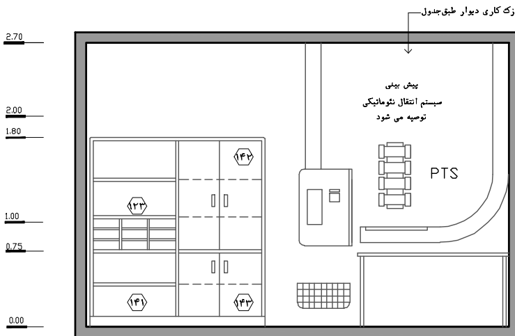
نقشه ۲-۵۳-۲- نمای ۲- مقیاس ۱:۵۰
