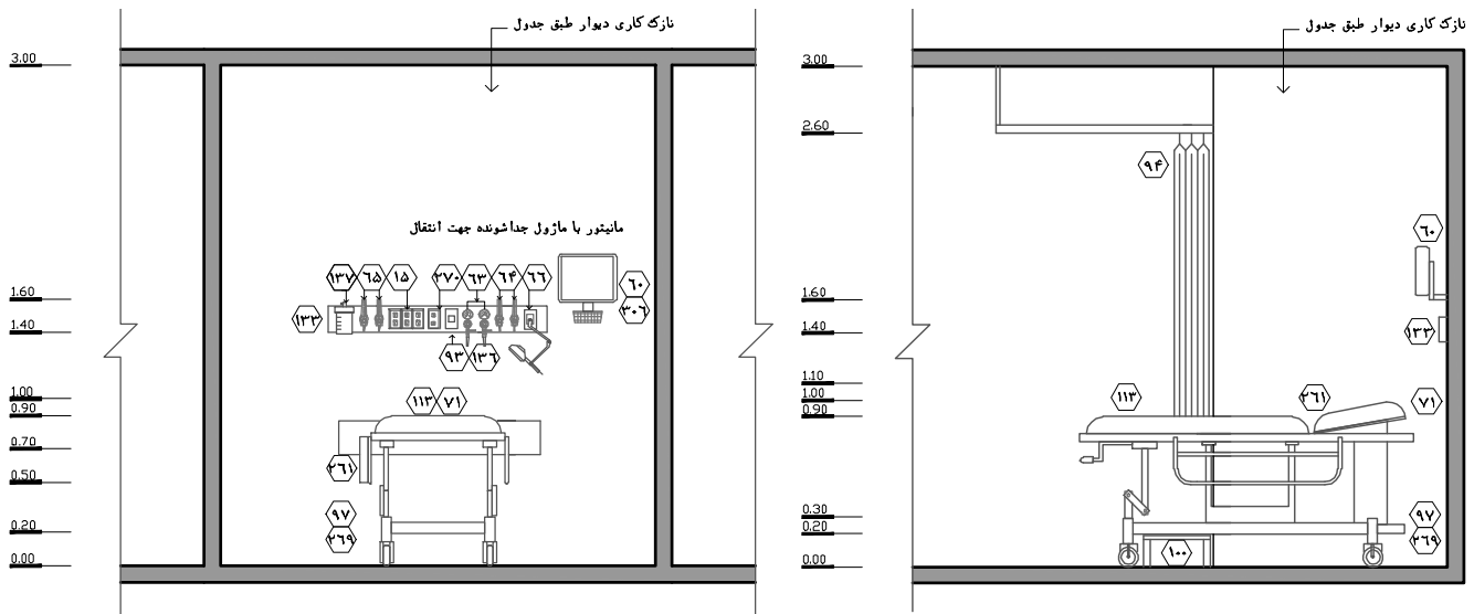
نقشه ۲-۴۶- نمای ۱- مقیاس ۱:۵۰
