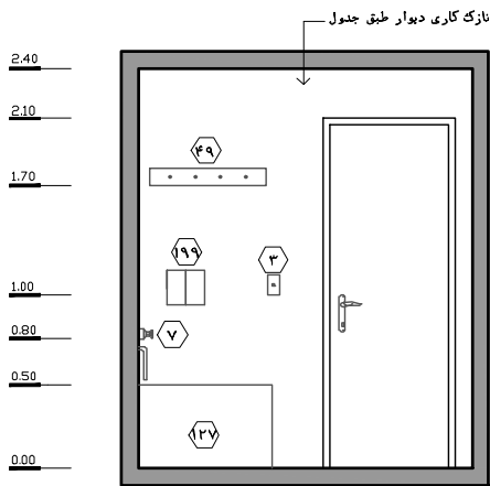
نقشه ۲-۲۲- نمای ۱- مقیاس ۱:۵۰
