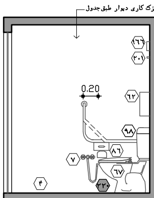
نقشه ۲-۶۴- نمای ۲- مقیاس ۱:۵۰
