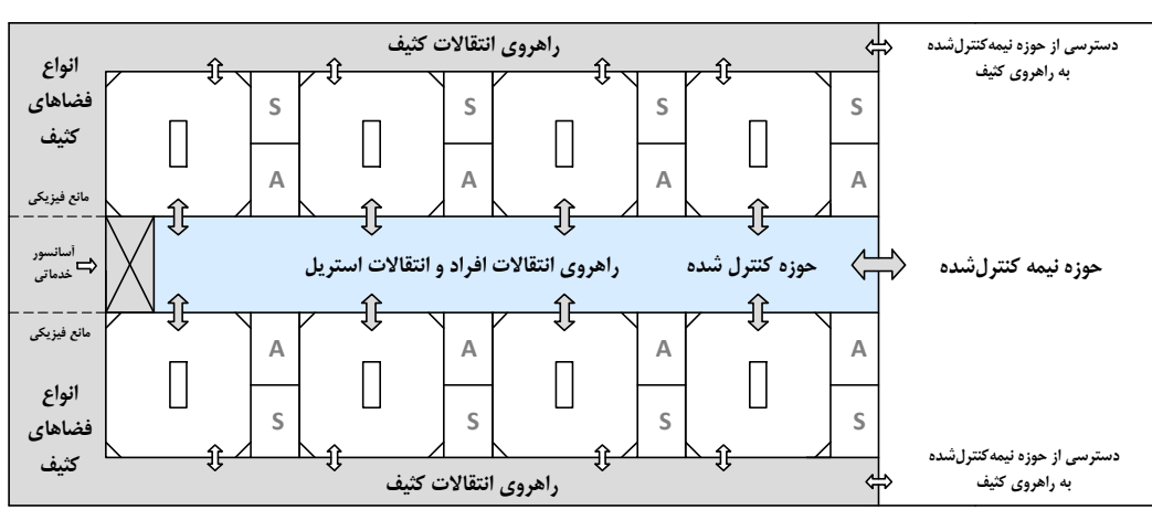
شکل ۲-۱۱- طراحی دو راهرویی با راهرو کثیف
