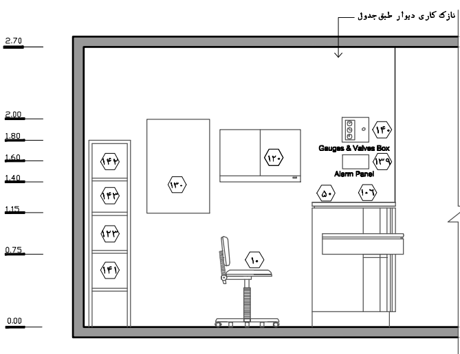
نقشه ۳-۵۴-۱- نمای ۳- مقیاس ۱:۵۰
