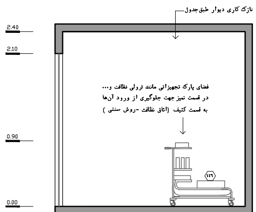
نقشه ۲-۳۸- نمای ۴- مقیاس ۱:۵۰
