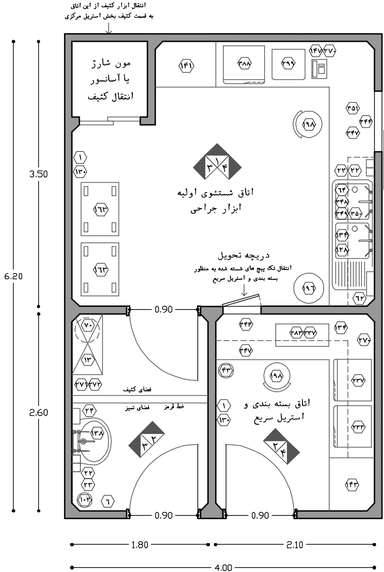
نقشه ۲-۷۷- پلان نمونه‌ای اتاق شستشوی ابزار و استریل سریع در بخش‌های اعمال جراحی کوچک و متوسط (تا ۹ اتاق عمل) - مقیاس ۱:۵۰
